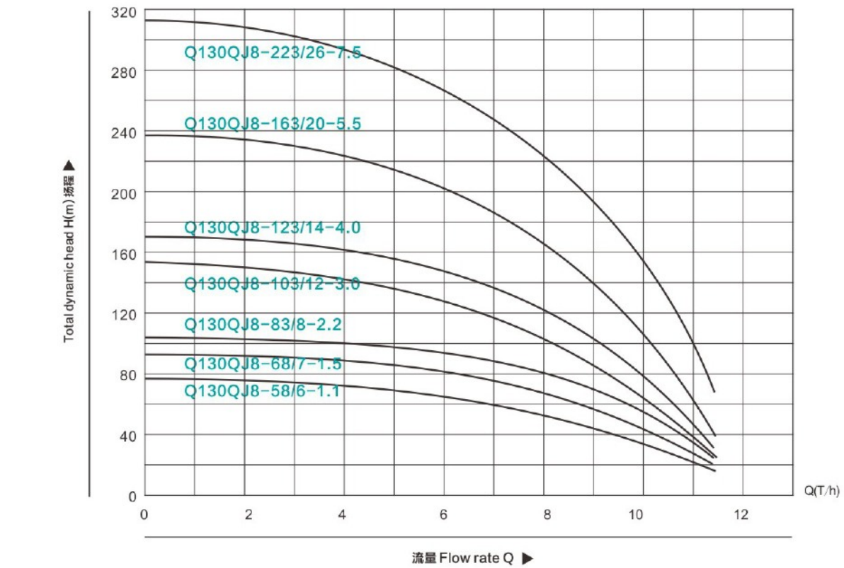
Q130JD-8T性能参数表 PERFORMANCE TABLE
